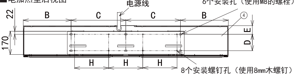
■电加热型后视图
