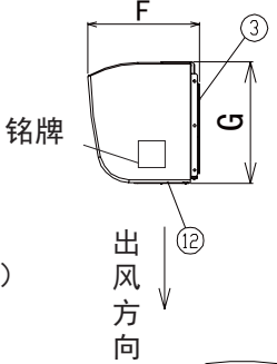
■电加热型右视图
